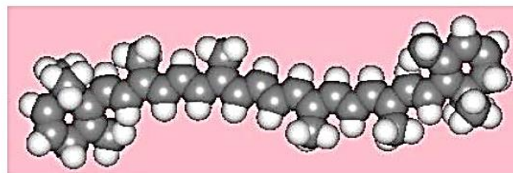
Carotène (rouge)
