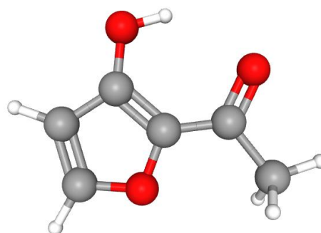
Isomaltol
