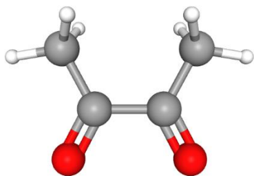
Diacetyl (butane-2,3-dione)
