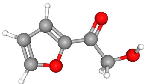
2(-2-hydroxyacetyl)-furan
