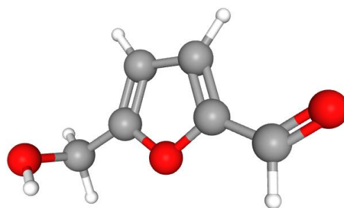
5-hydroxyméthyl-furfural
