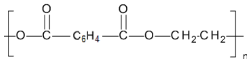
PET Polyéthylène téréphtalate
