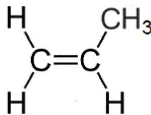
Propylène
