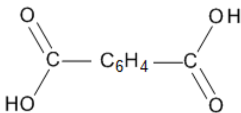
Acide téréphtalique
