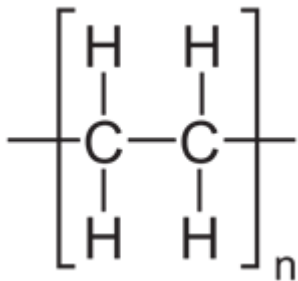
PE polyéthylène
