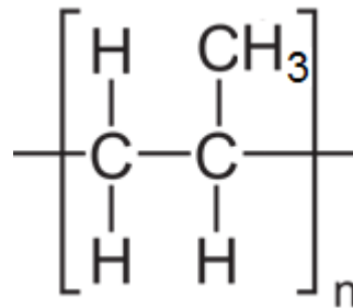
PP polypropylène
