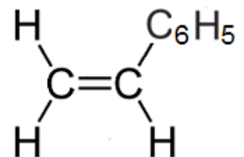
Styrène
