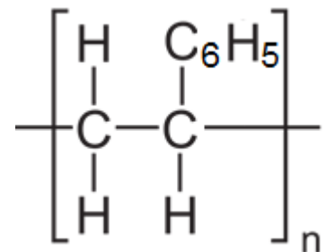
PS polystyrène
