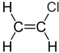
Chlorure de vinyle
