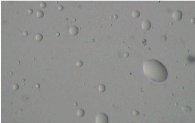
Gouttes d'huile en suspension dans l'eau
