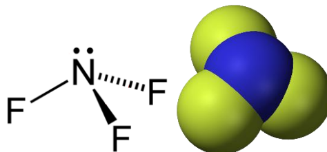
trifluorure d'azote, \text{NF}_3
