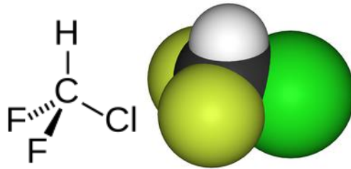
chlorodifluorométhane, \text{CHClF}_2
