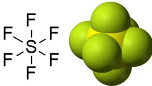
hexafluorure de soufre, \text{SF}_6
