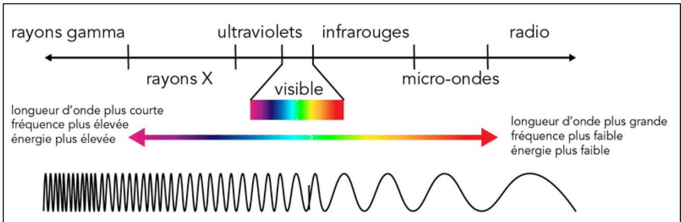
Image 2 : Le spectre électromagnétique (source : NASA)
