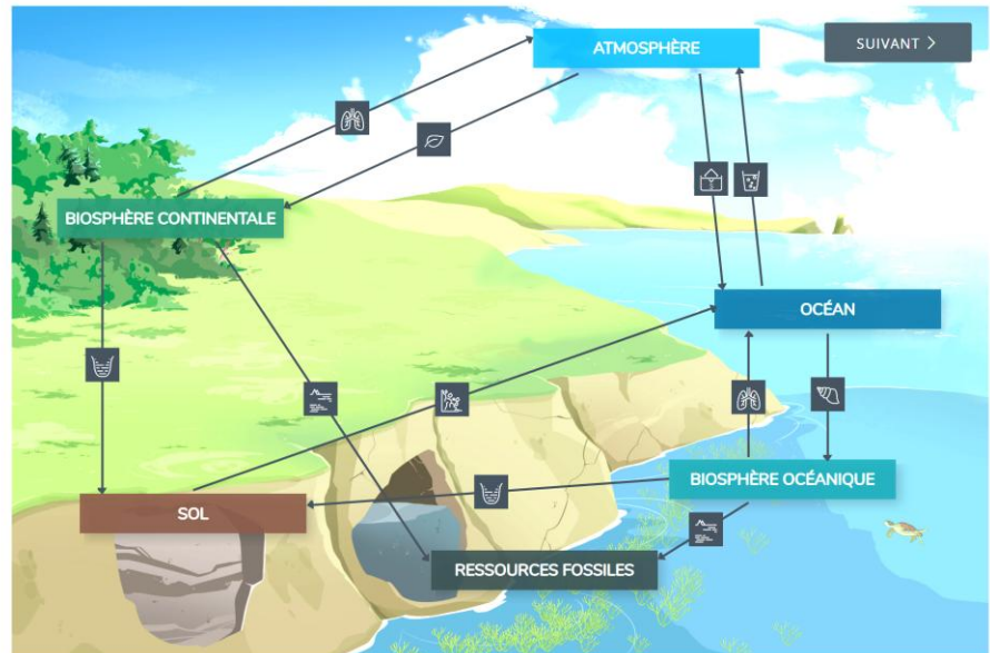
LE CYCLE NATUREL DU CARBONE
