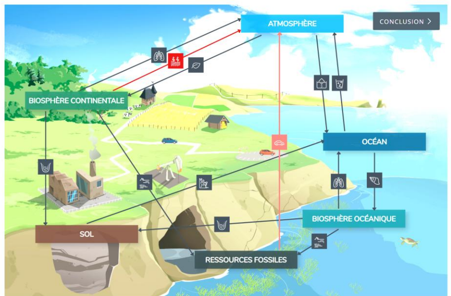
LE CYCLE DU CARBONE À L'HEURE ACTUELLE
